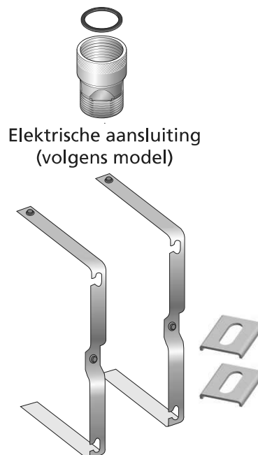
Bevestigingsbeugels (horizontaal)
