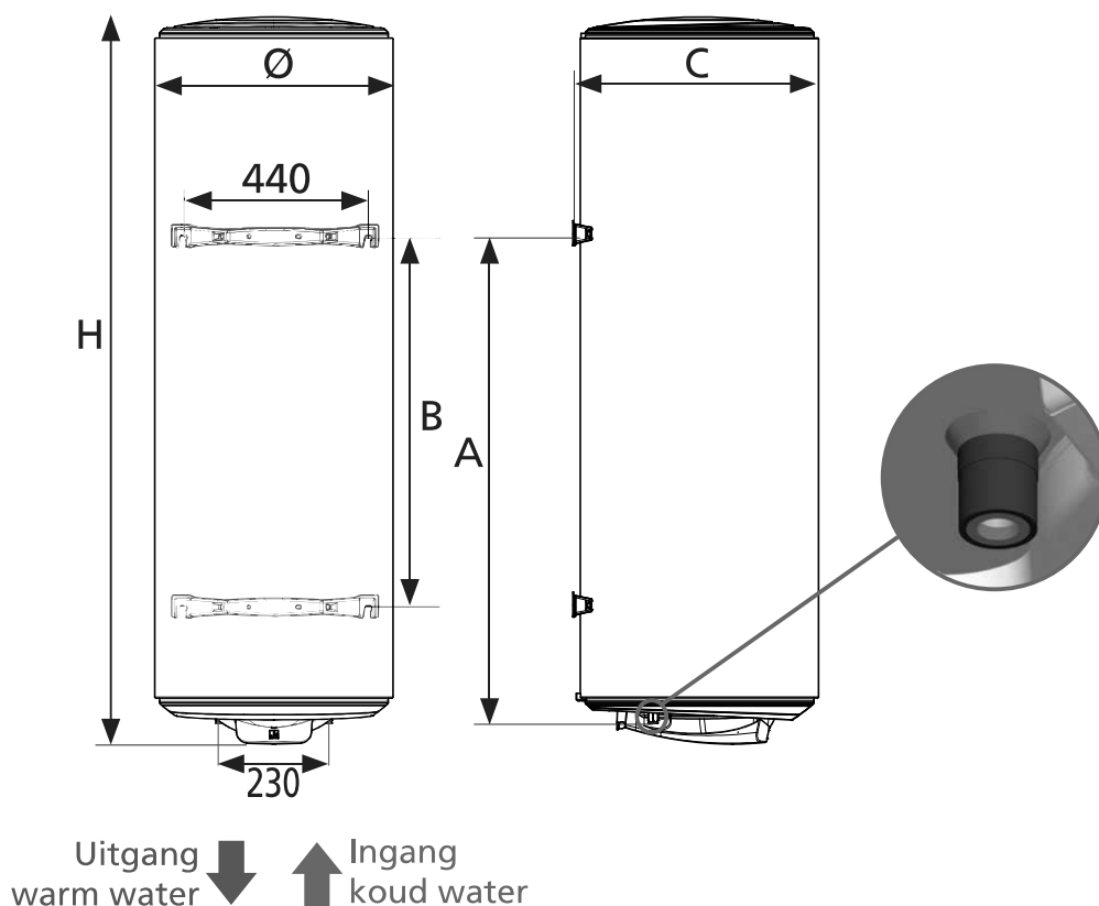
Schematische weergave
